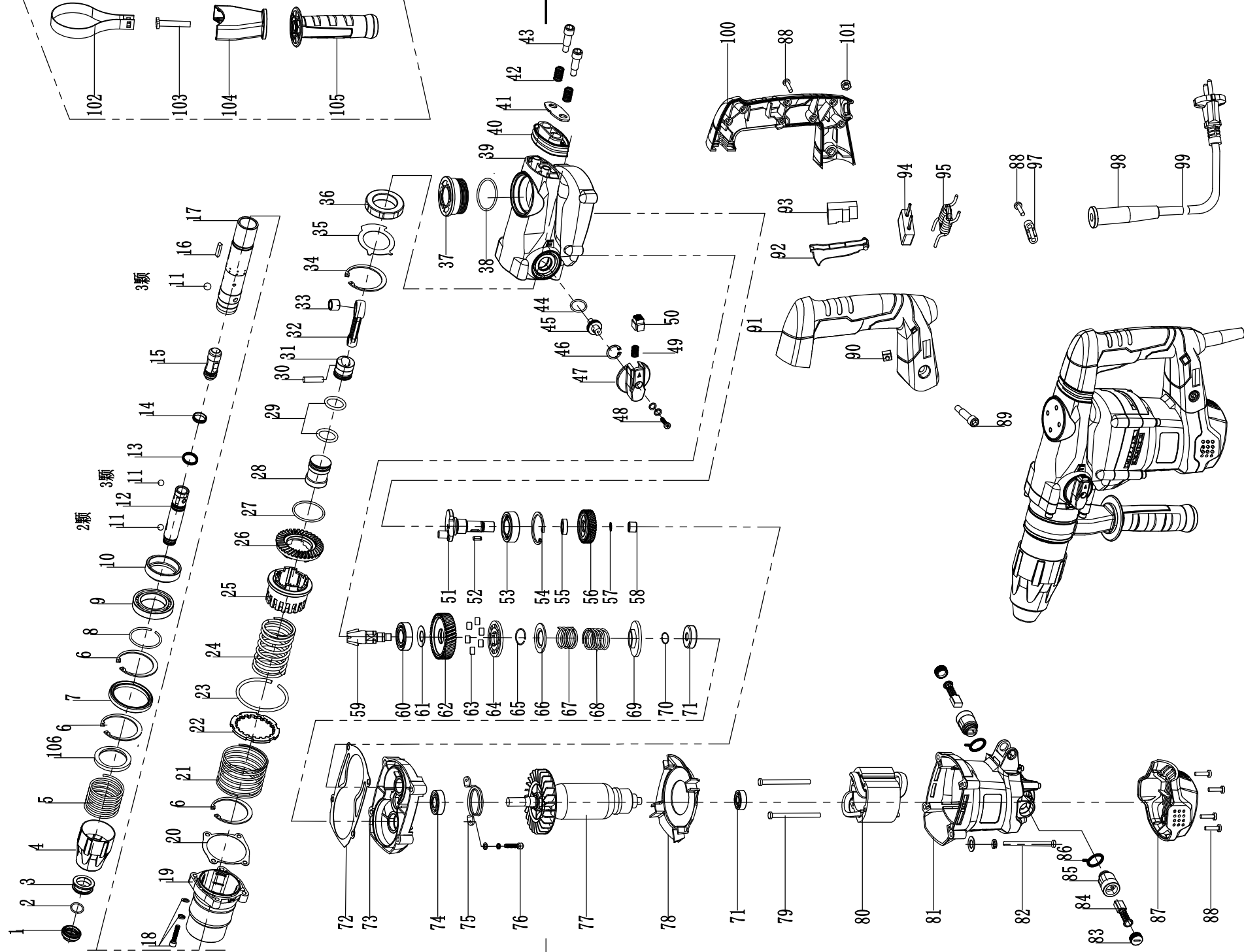
DC42KA爆炸图 (橡胶头、钢柱脱扣、带调速)
